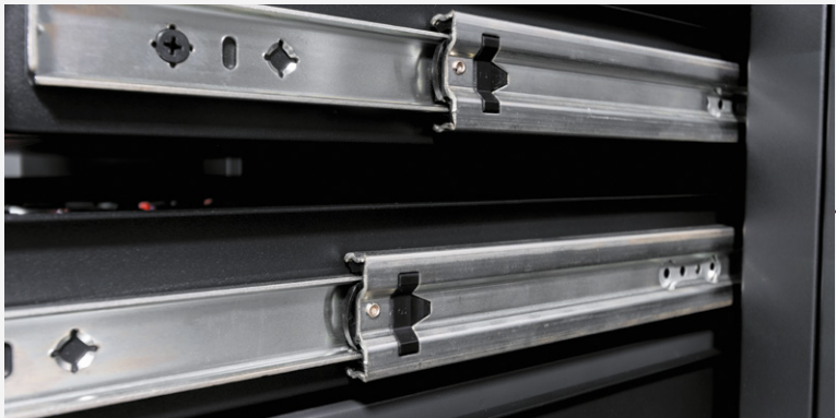
Glissières à billes pour tiroirs Tous les tiroirs sont équipés de glissières à billes, ce qui leur permet de s'ouvrir et de se fermer en douceur et en silence, tout en offrant une grande capacité de charge.
